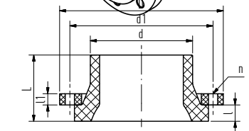
SDR 6 / 7.4 / 9 / 11 / 17.6
